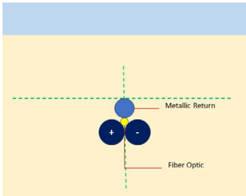
Figuur 2-3 Ingegraven kabelbundel
