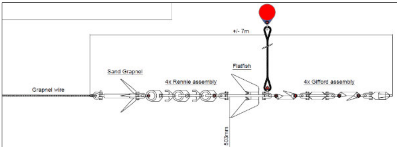
Figuur 4-4: Voorbeeld van grapneltrein
