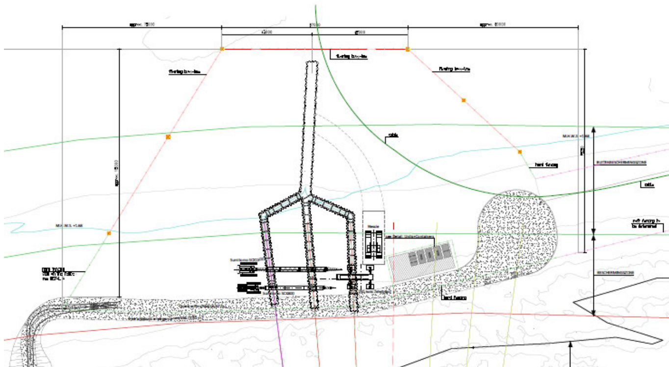
Figuur 3-7 Inrichting werkterrein strand, de complete inrichtingstekening is als Bijlage I aan het werkplan toegevoegd.
