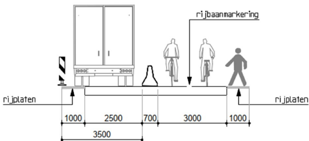
Figuur 3-5 Indeling onderhoudsweg Veerse Gatdam (incl. barrier)
