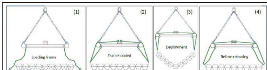
Figuur 4-11: Schematische weergave van matrasininstallatie
