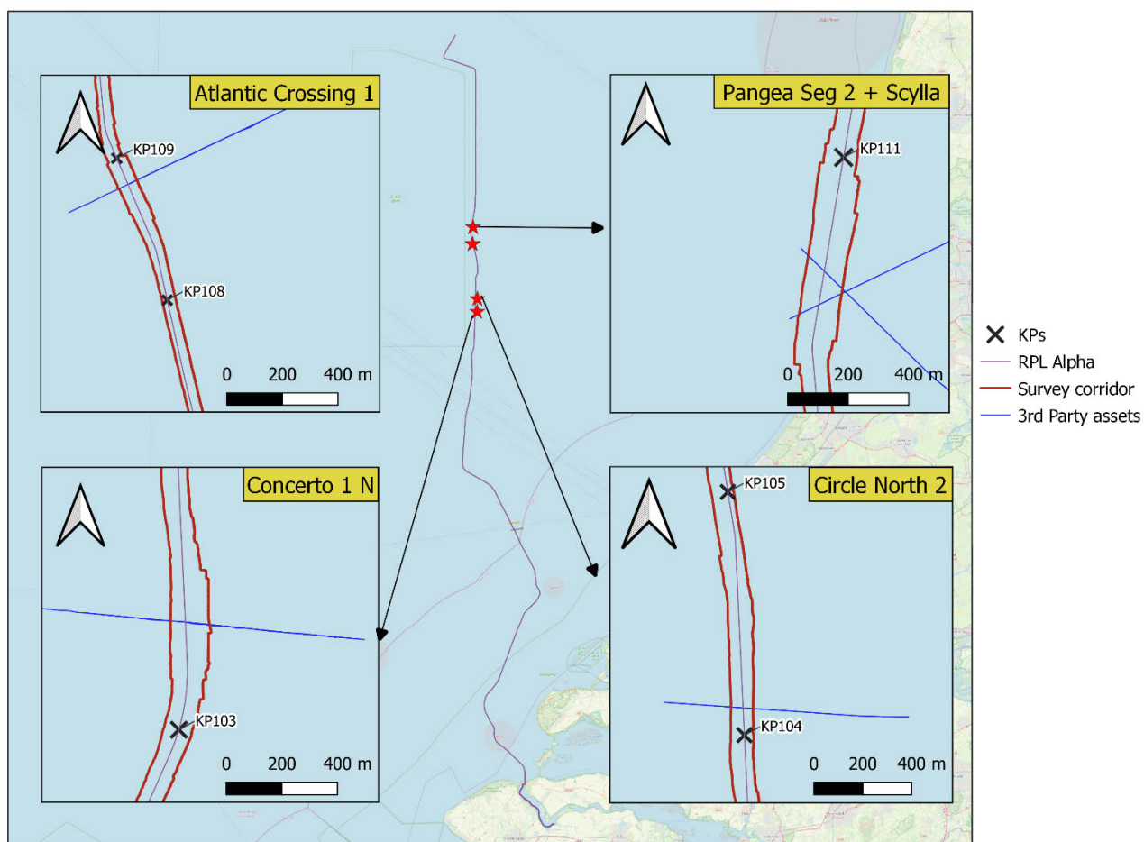
Figuur 2-8 IJmuiden Ver Alpha – Kruisingen met bestaande infrastructuur (2)
