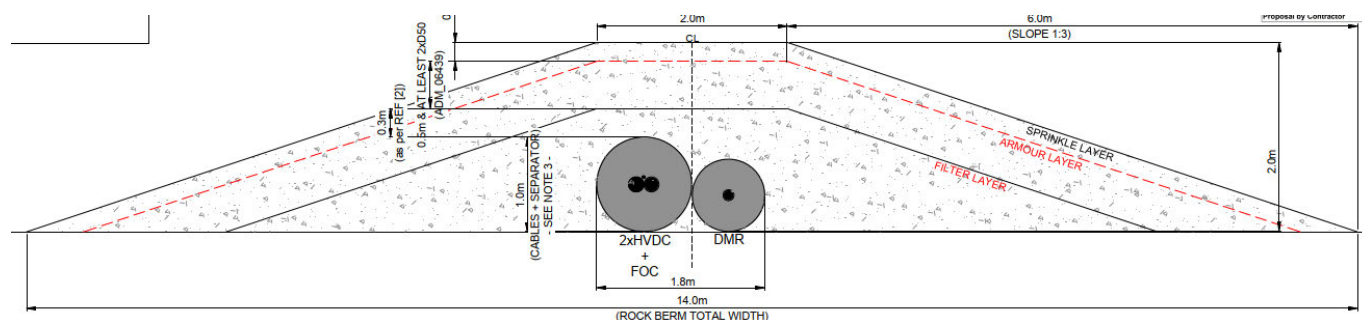
Figuur 4-26 Dwarsdoorsnede ontwerp kabelkruising
