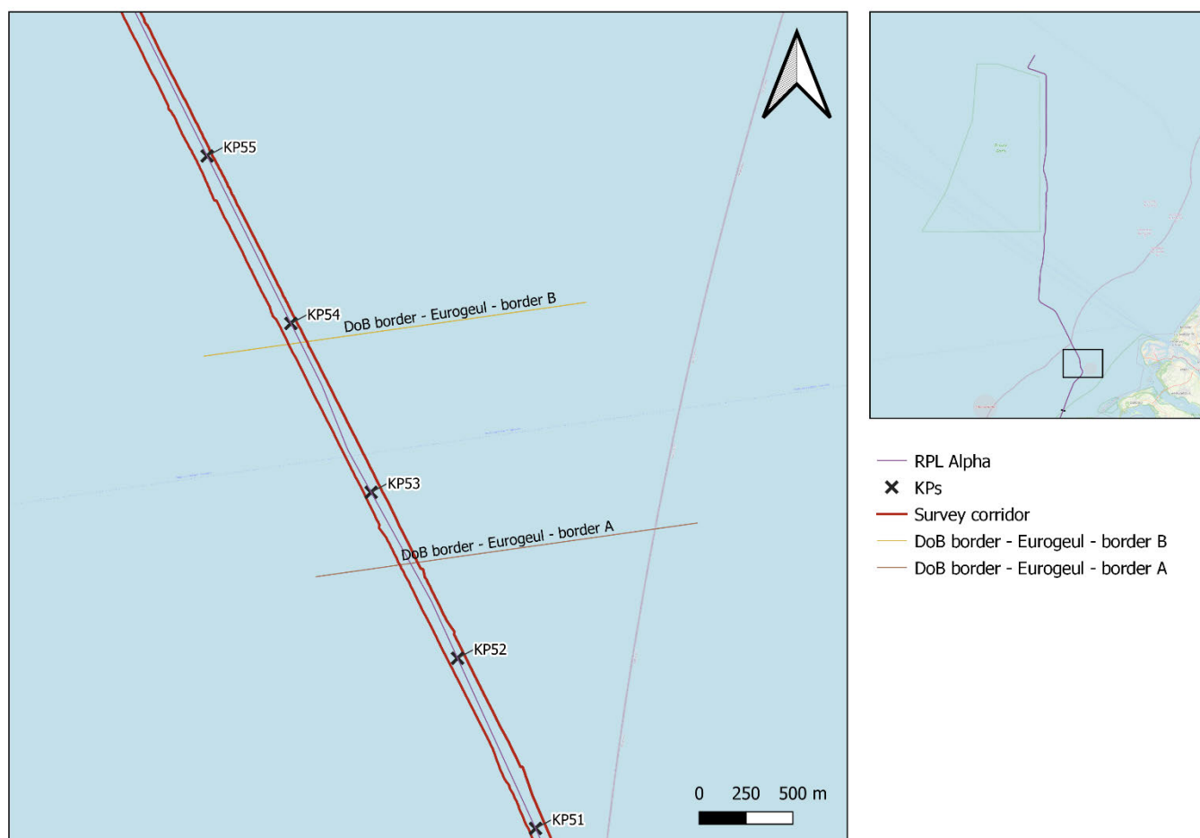
Figuur 2-9 Kruising met Eurogeul
