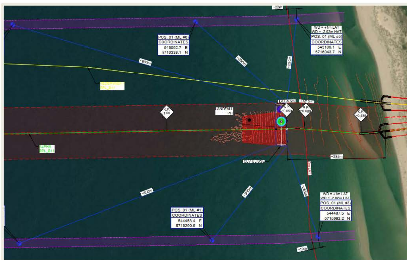
Figuur 3-18 Overzicht ankerpatroon
