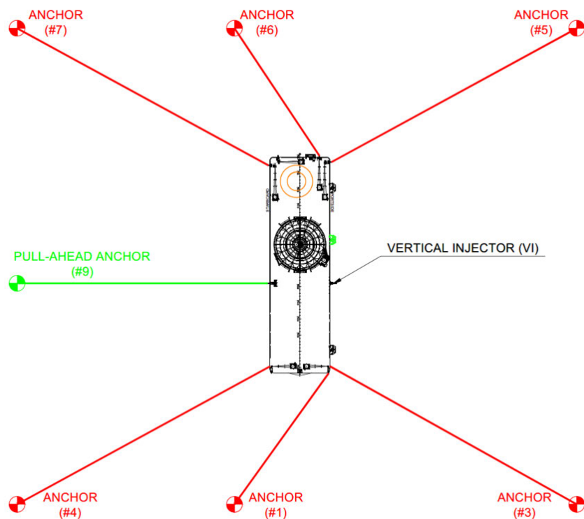
Figuur 3-16 Ankersysteem
