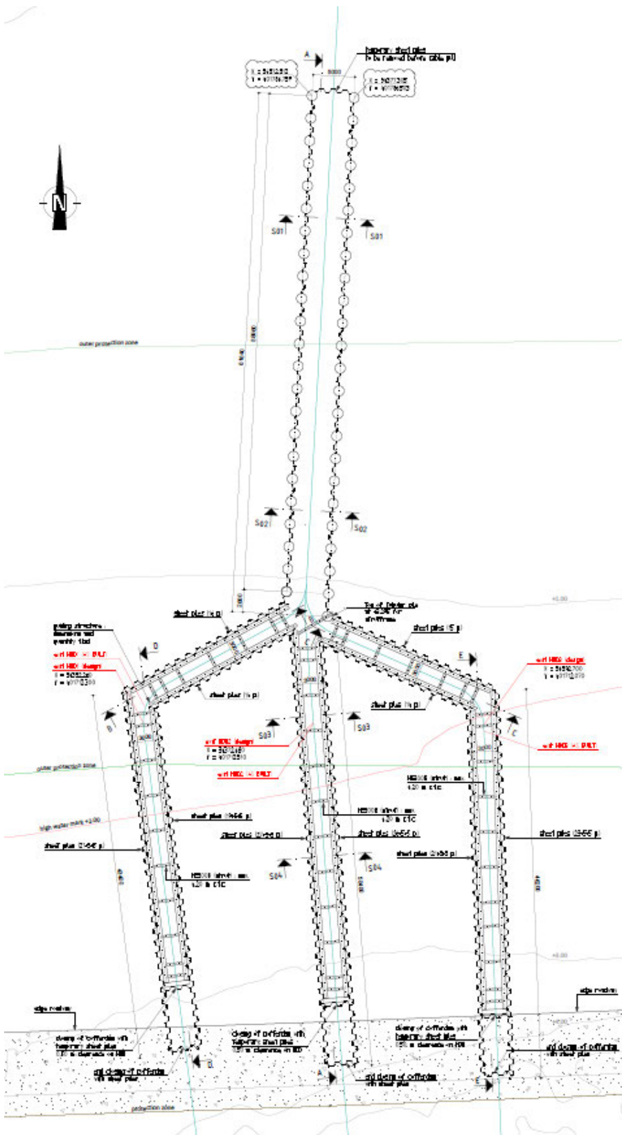
Figuur 3-8 Bovenaanzicht ontwerp kofferdammen (zuidzijde, drietand) en combiwand (noordzijde, enkel), de ontwerpdocumenten zijn als Bijlage J1 aan het werkplan toegevoegd.
