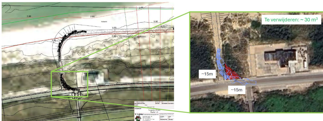
Figuur 3-6 Bochtverflauwing dijkopgang voormalig strandpaviljoen View
