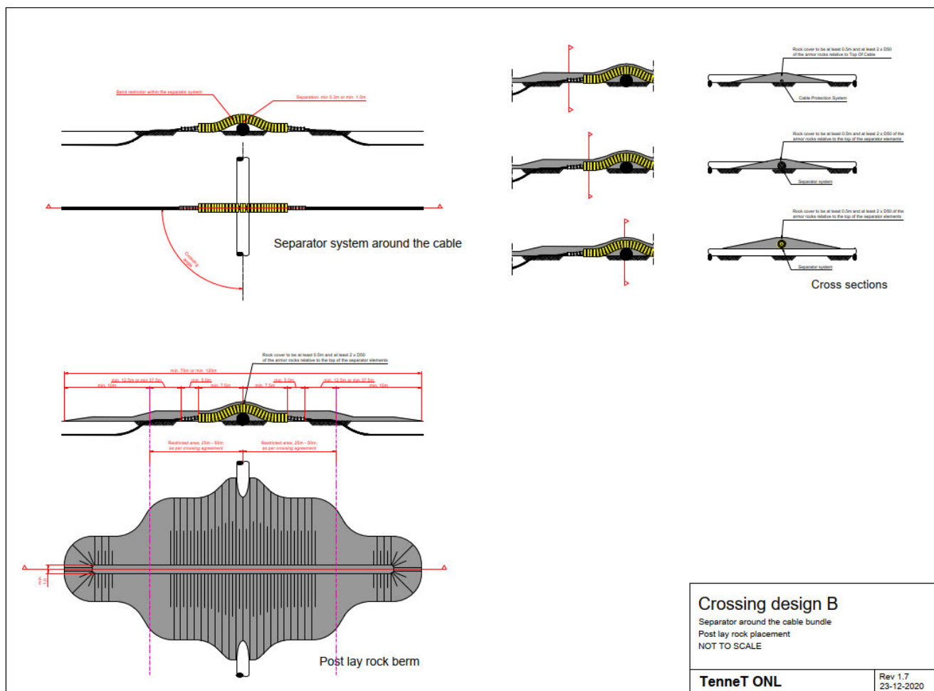
Figuur 4-8: Voorlopig ontwerp van een kruising met scheidings-CPS
