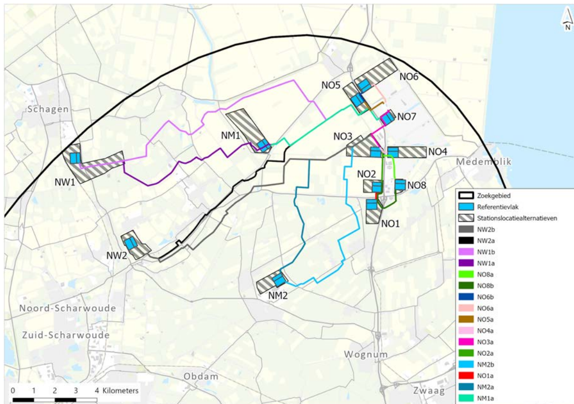
Afbeelding 4.3 Alternatieven noordelijk 380/150 kV-hoogspanningsstation met referentievlakken en alternatieven ondergrondse 150 kV-verbinding
