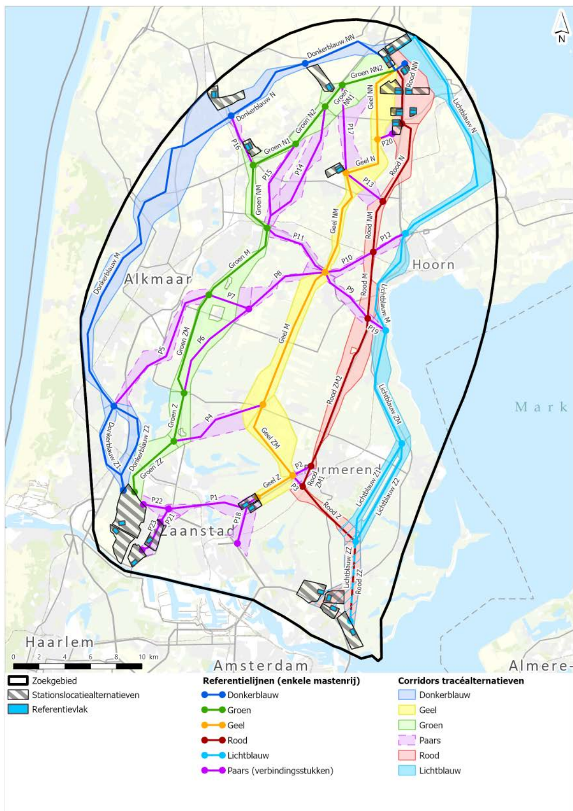
Afbeelding 3.3 De alternatieven voor de hoogspanningsverbinding en -stations op de kaart. De verbindingsstukken zijn paars
