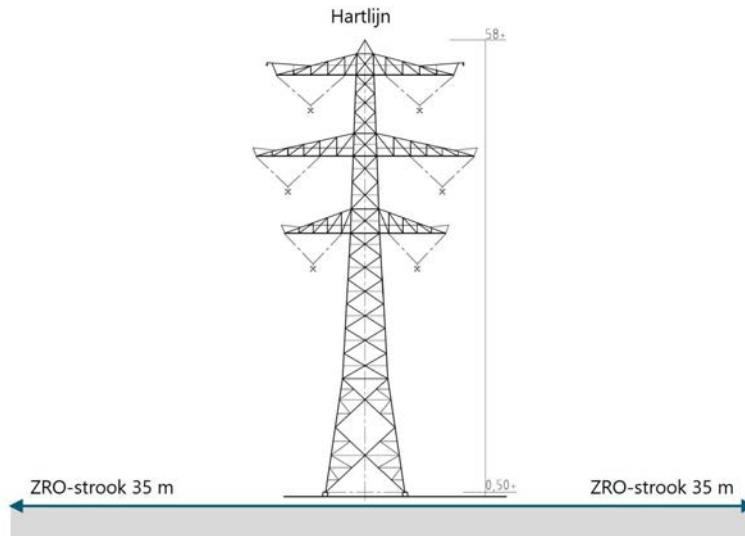
Afbeelding 3.1 Een schematische weergave van een hoogspanningsmast, inclusief de ZRO-strook
