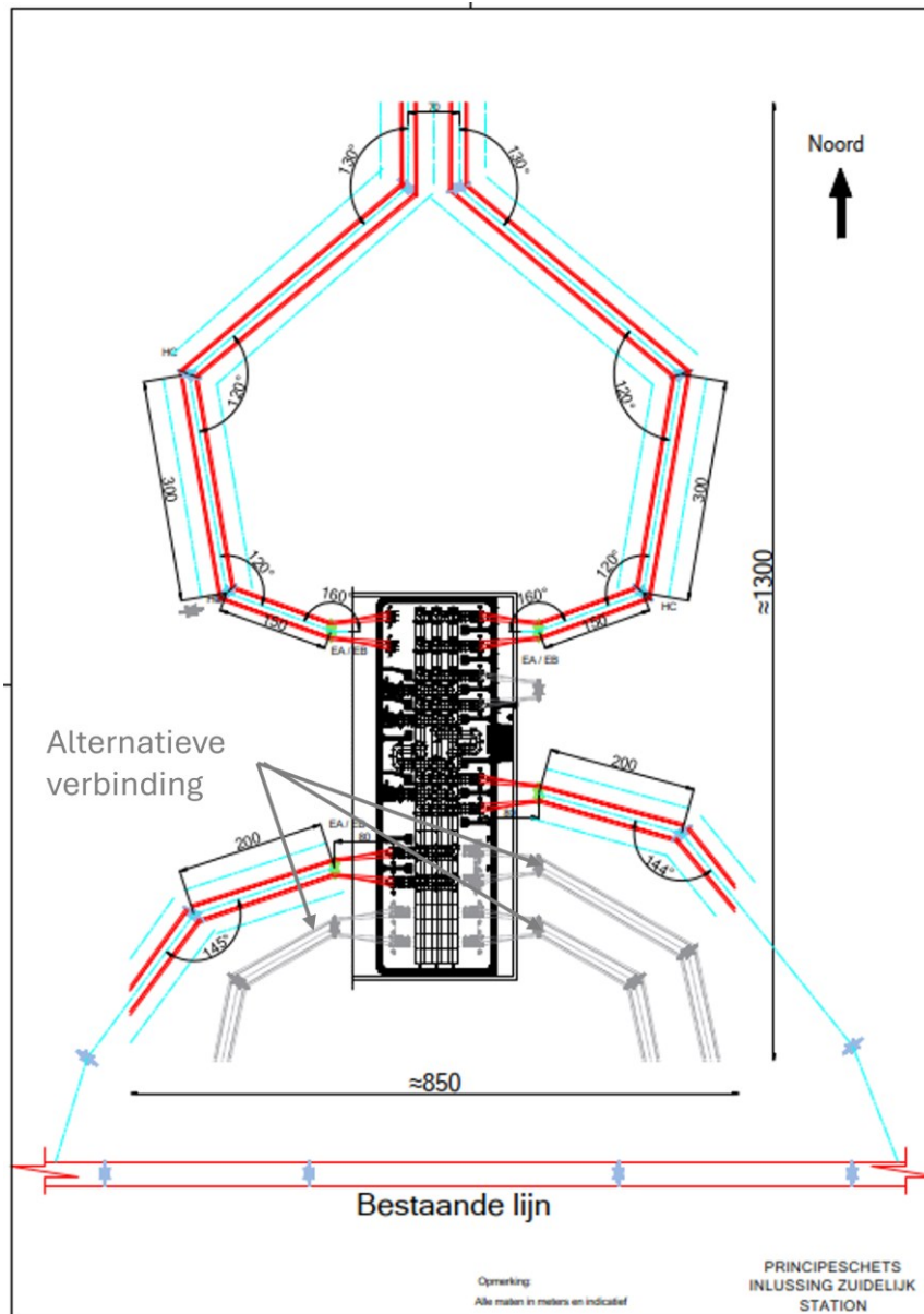
Afbeelding 6.9 Voorbeeld 3, inlussing 380 kV zuidelijk station
