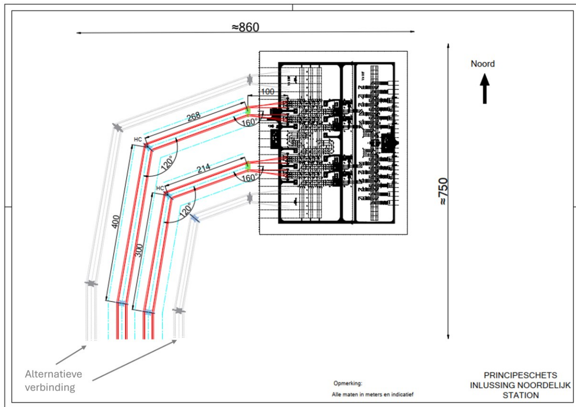
Afbeelding 6.4 Voorbeeld 2, inlusing 380/150 kV noordelijk station
