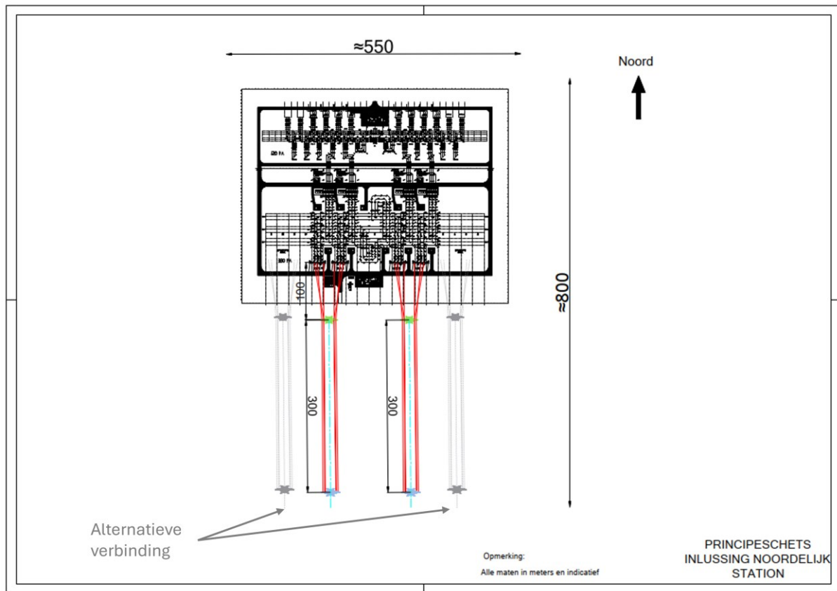
Afbeelding 6.3 Voorbeeld 1, inlussing 380/150 kV Noordelijk station
