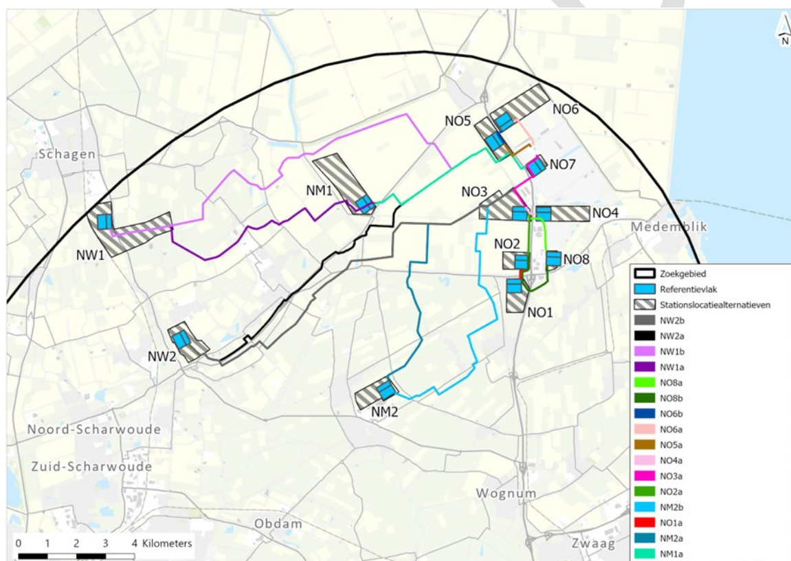
Afbeelding 5.8: Alternatieven noordelijk 380/150 kV-hoogspanningsstation met referentievlakken en alternatieven ondergrondse 150 kV-verbinding
