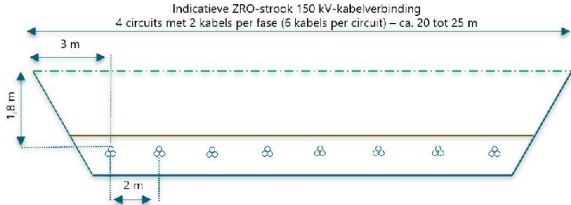
Afbeelding 3.9 Indicatieve ZRO-strook 150 kV-kabelverbinding (eigen afbeelding)
