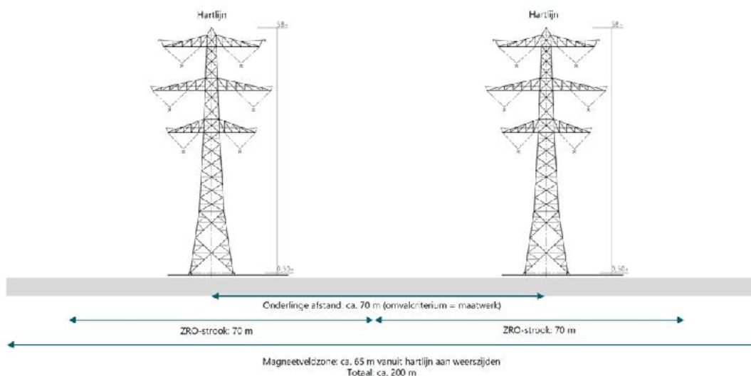
Afbeelding 1.5 Doorsnede van de benodigde ruimte bij twee mastenrijen (masttype Moldau)
