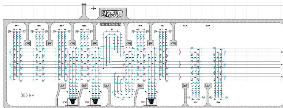
Afbeelding 5.3 Onderdelen 380 kV-hoogspanningsstation
