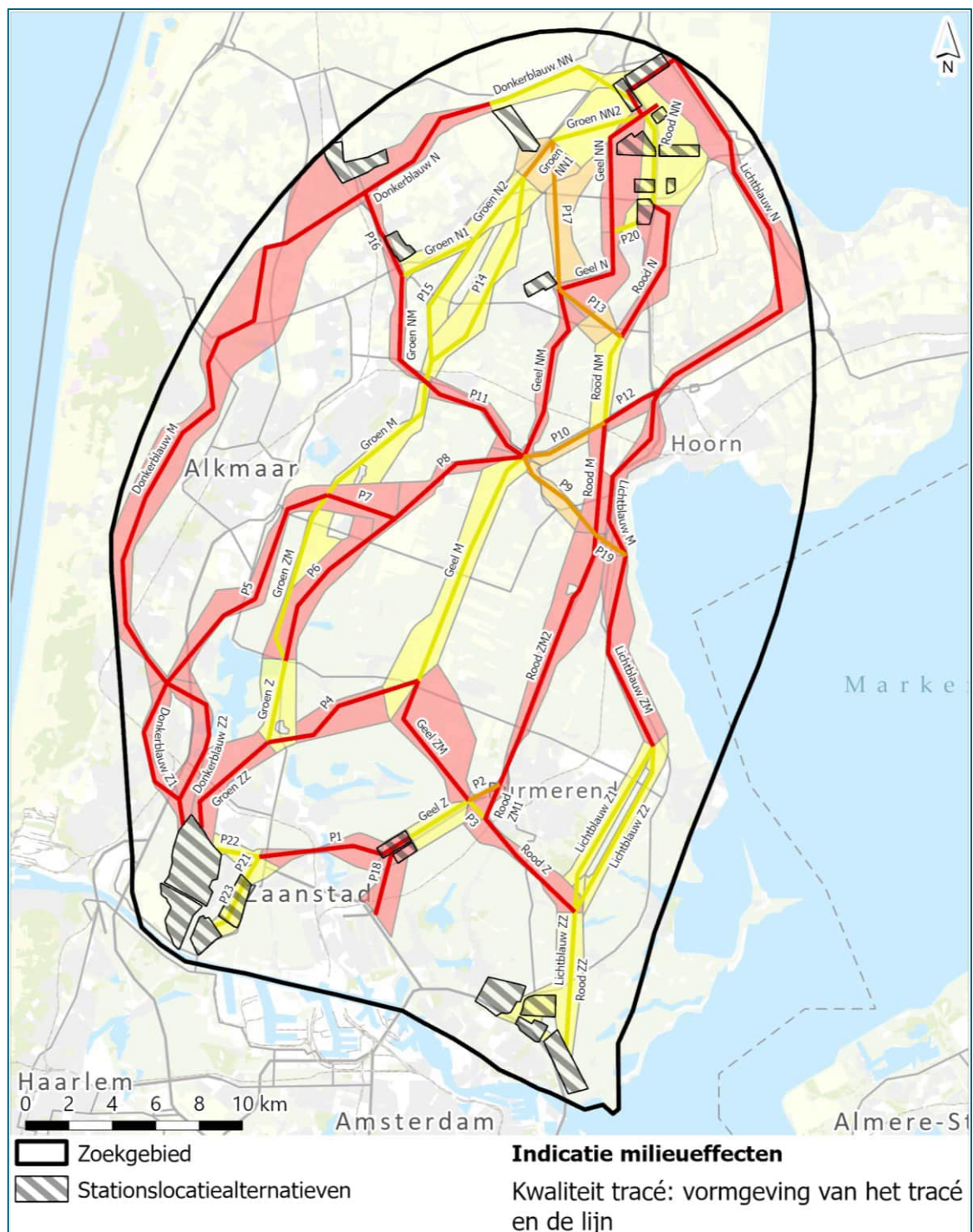
Afbeelding 6.10 Effectbeoordeling kwaliteit tracé: vormgeving van het tracé van de lijn voor een dubbele 380 kV-mastenrij
