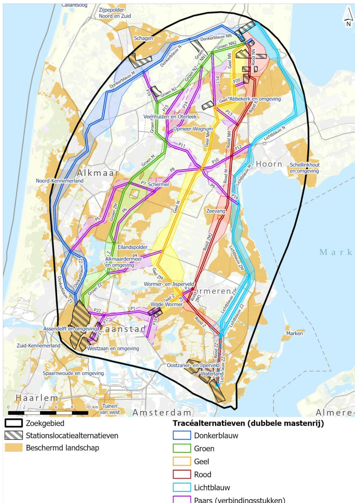
Afbeelding 6.11 Beïnvloeding van de gebiedskarakteristieken - 380 kV-tracéalternatieven met dubbele mastenrij
