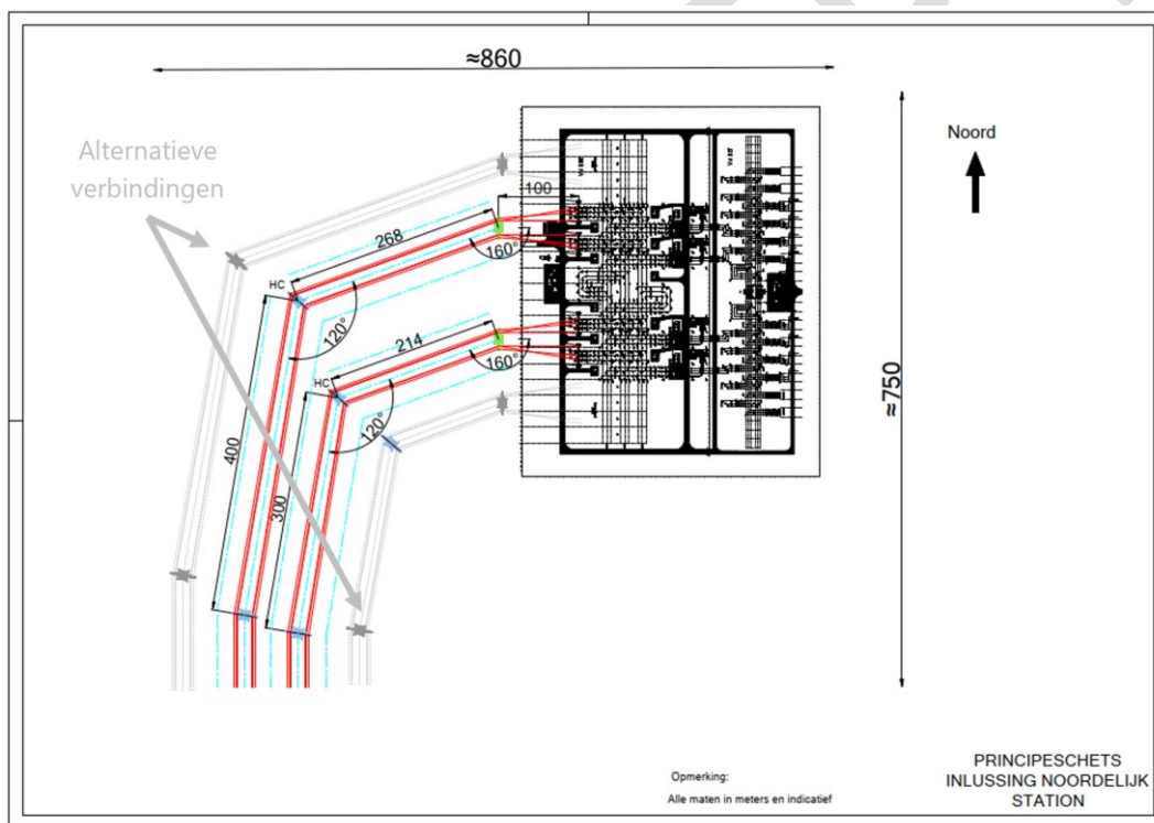
Afbeelding 4.3 Opstelling 2, indicatieve weergave 380/150 kV-station
