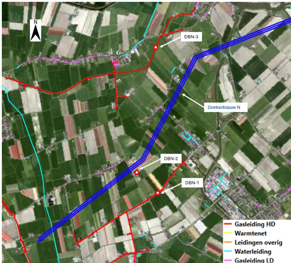
Afbeelding I.5 Knelpunten parallelligging deeltracé donkerblauw N
