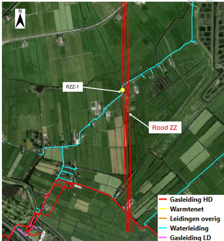
Afbeelding IV.1 Knelpunten parallelligging deeltracé rood ZZ
