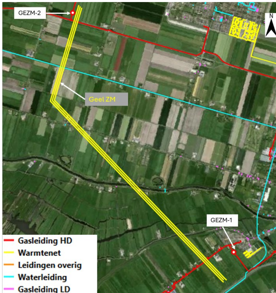
Afbeelding III.2 Knelpunten parallelligging deeltracé geel ZM
