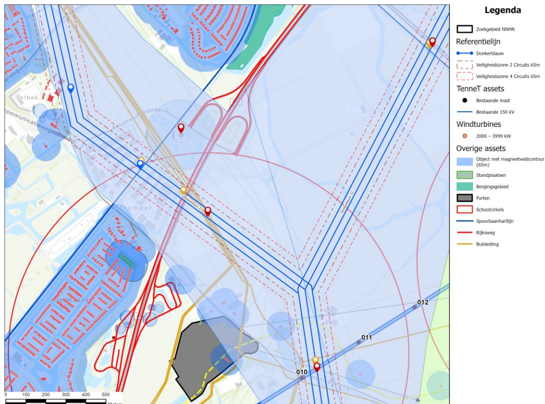
Afbeelding 5.4 Voorstelling knelpunt 12130
