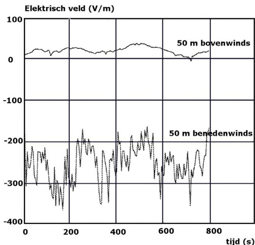
Figuur 8 Meting van het elektrische veld aan het aardoppervlak boven- en benedenwinds van een bovengrondse 400 kV hoogspanningslijn (bron: Fewes et al [29])
