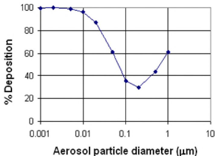
Figuur 1: Totale depositie van ingeademde fijn stof deeltjes in de long, indien er geen elektrische opladingseffecten zijn (ICRP 66 long model)
