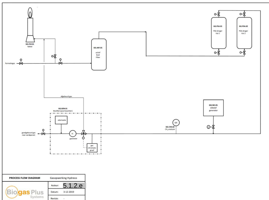
Figuur 3.3: PFD van de opwaarderingsunit
