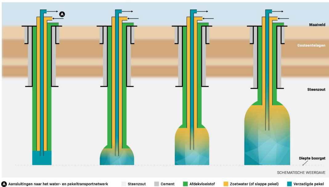
Figuur 10: Schematische weergave van caverneontwikkeling door de tijd heen.
