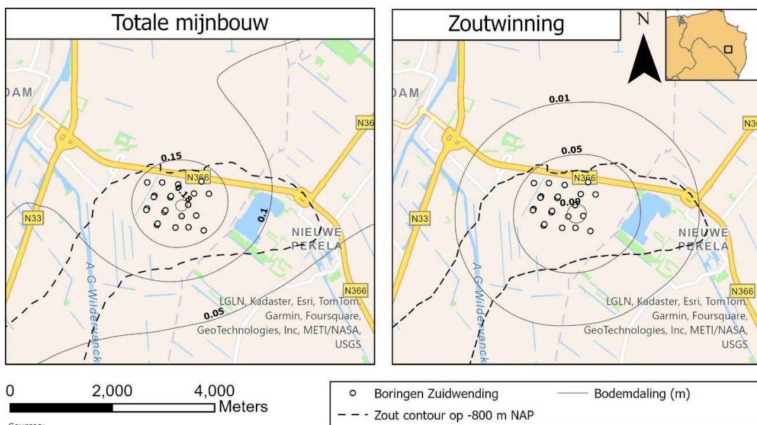
Figuur 13: Bodemdalingssprognose 2025; verwacht scenario.
