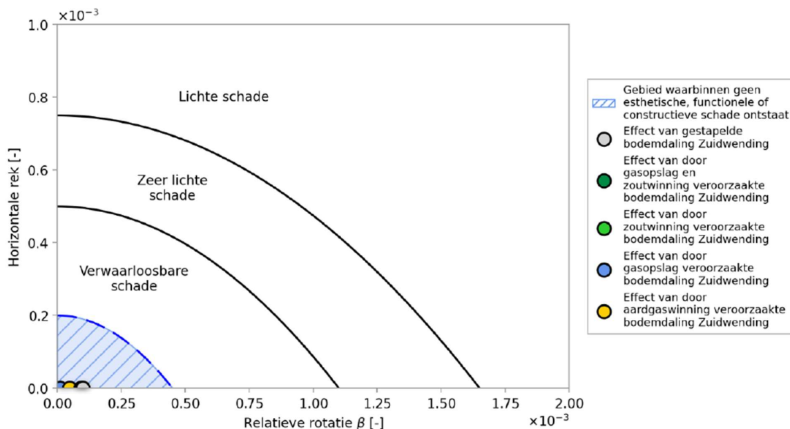
Figuur 31: Grenswaarden voor schade als gevolg van bodemdaling en berekende waarden Zuidwending
