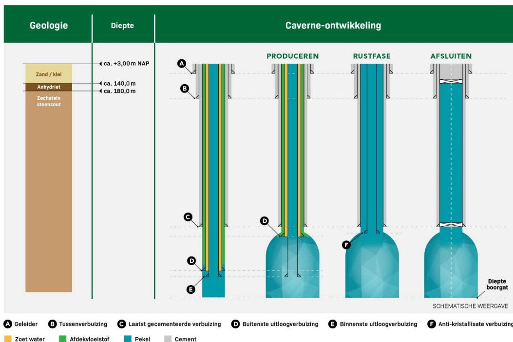
Figuur 8: Generiek verbuizingsschema tijdens verschillende fases van caverneoperatie
