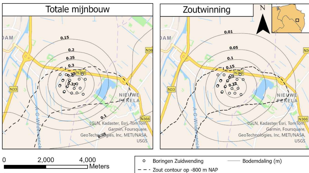
Figuur 17: Bodemdalingsprognose 2075; verwacht scenario.
