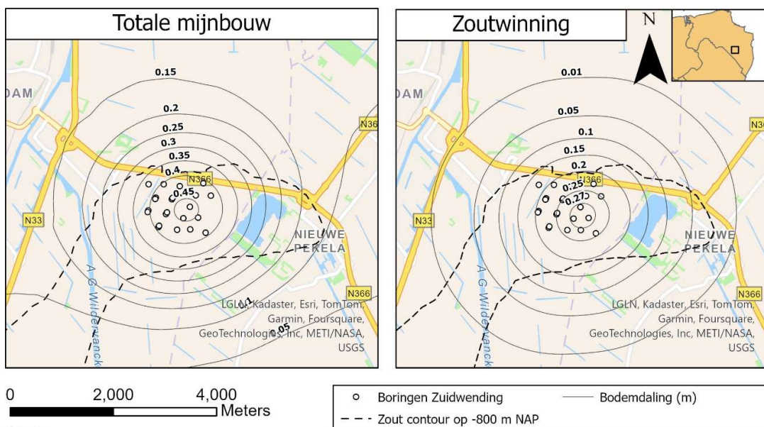
Figuur 21: Bodemdalingsprognose 2125; verwacht scenario.
