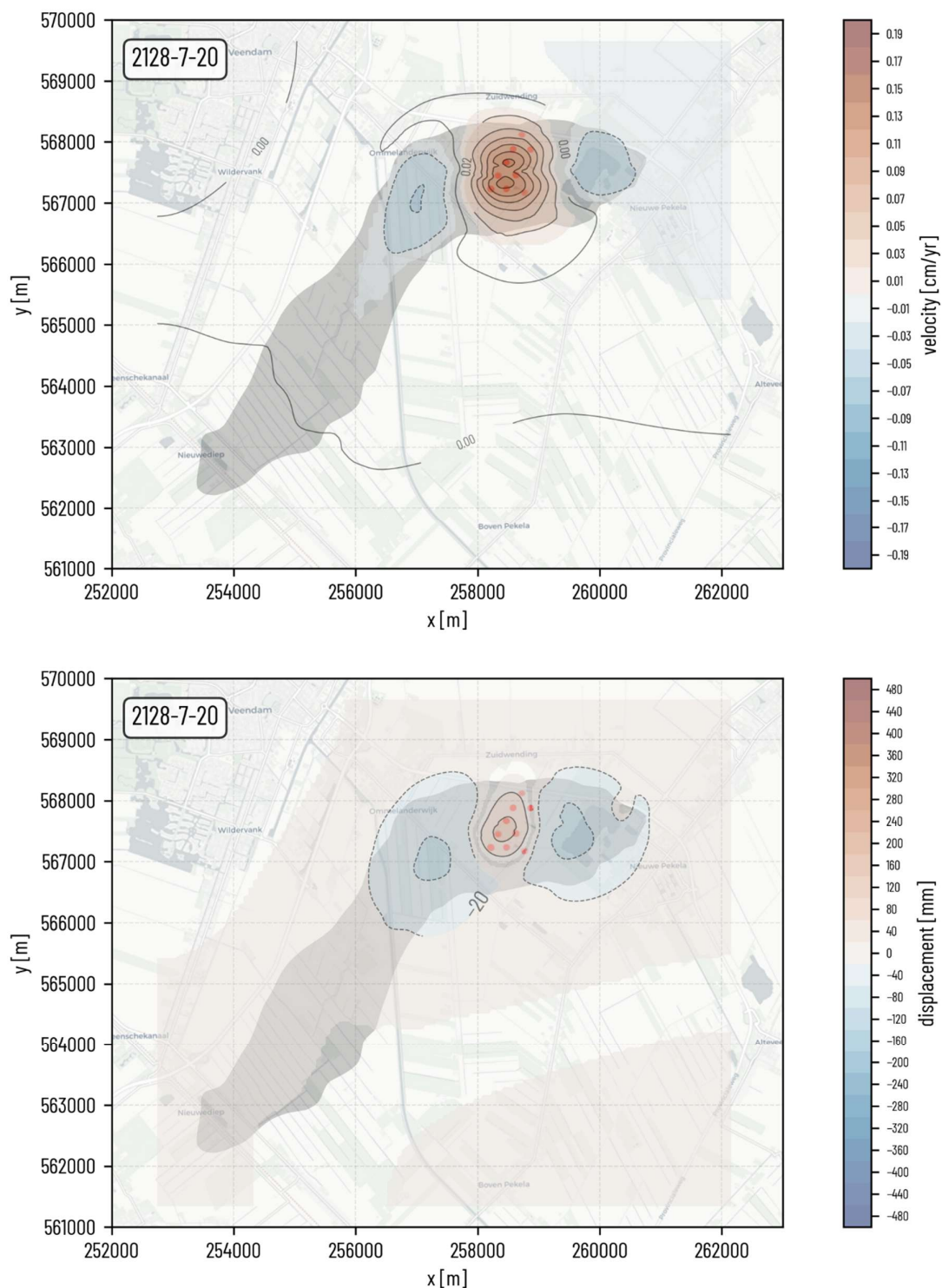
Figuur 29: Voorbeeld van bodemdalingsprognoses uit het deterministische (3D) model voor het jaar 2128, (CCC 2024). Het figuur boven laat de bodemdalingsnelheid zien, onder de totale bodemvervorming (daling in blauw, stijging in rood). In deze versie van het model is bewust geen rekening gehouden met de gasopslag cavernes om zo de effecten van de zoutwinningscavernes in dit winningsplan te zien. Effecten van gaswinning (op basis van NAM prognose 2080) zijn wel meegenomen. Voor de versie met gasopslagcavernes zie het CCC rapport.
