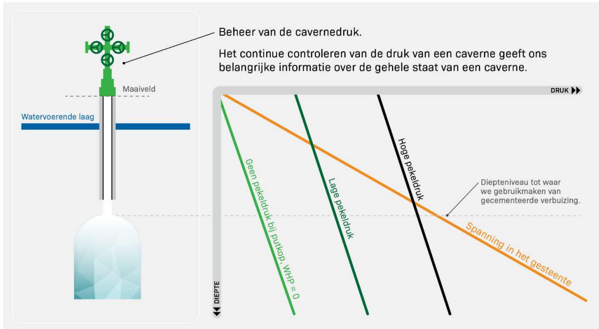
Figuur 6: schematische weergave van pekeldruk in een caverne in relatie tot de druk die gemeten wordt aan het maaiveld. Spanning in het gesteente is indicatief voor de onverstoorde situatie zonder dat er een caverne is, ofwel het "far field" spanningsveld. Door de aanwezigheid van de caverne zelf zal de lijn anders lopen in de buurt van de caverne, en kan ook veranderen als gevolg van de druk in de caverne zelf.
