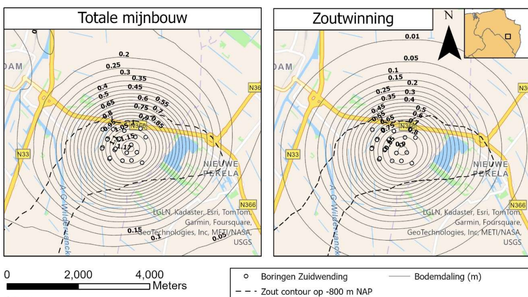
Figuur 26: Bodemdalingsprognose 2200, conservatief scenario
