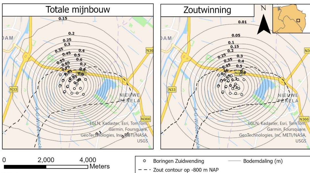
Figuur 24: Bodemdalingsprognose 2150, conservatief scenario
