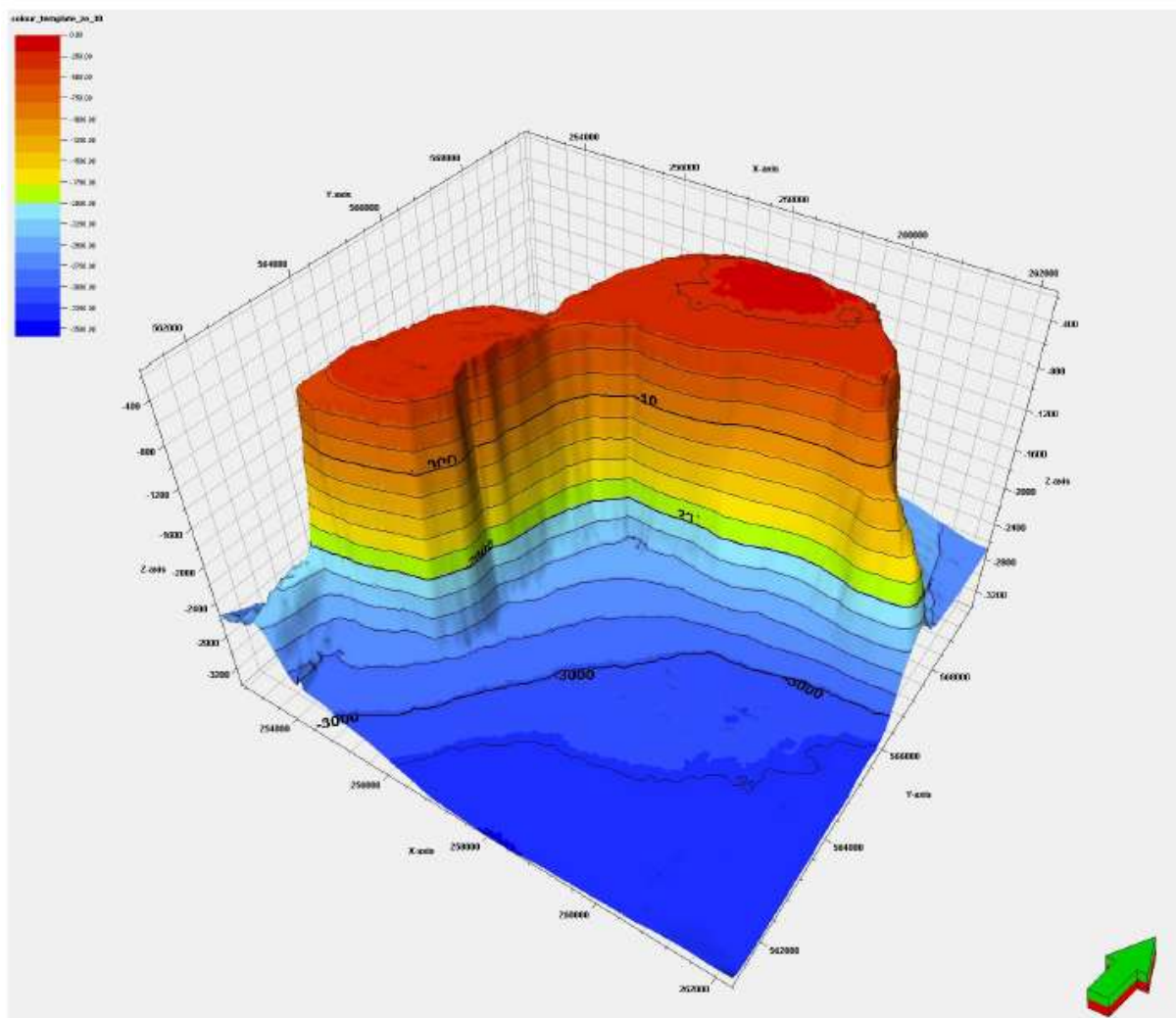
Figuur 4: 3D-weergave van de zoutpijl bij Zuidwending. Bron: TNO (via nlog.nl/steenzout )
