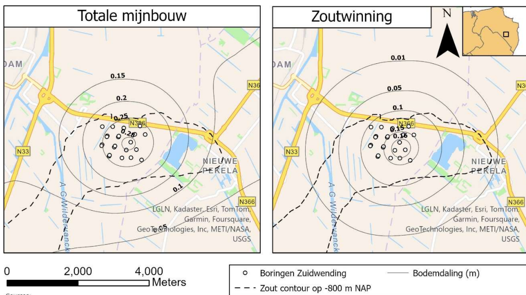
Sources: DEEP.KBB, 2024 Figuur 15: Bodemdalingsprognose 2050; verwacht scenario.
