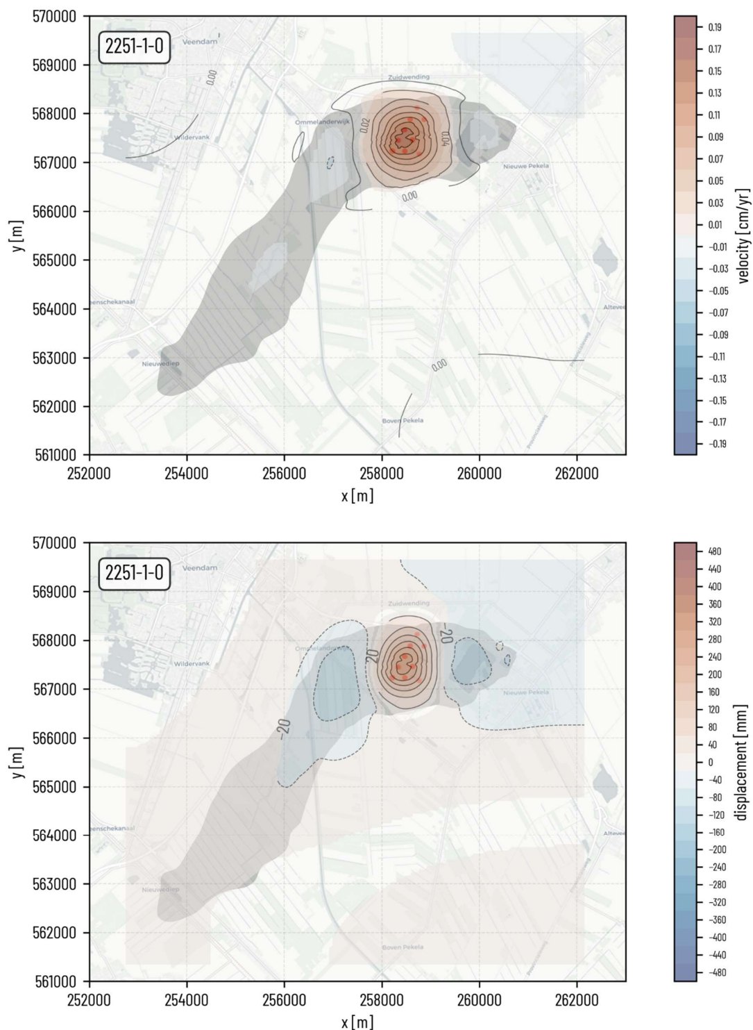
Figuur 30, Voorbeeld van bodemdalingsprognoses uit het deterministische (3D) model voor het jaar 2251, (CCC 2024). Het figuur boven laat de bodemdalingssnelheid zien, onder de totale bodemvervorming (daling in blauw, stijging in rood). In deze versie van het model is bewust geen rekening gehouden met de gasopslag cavernes om zo de effecten van de zoutwinningscavernes in dit winningsplan te zien. Effecten van gaswinning (op basis van NAM prognose 2080) zijn wel meegenomen. Voor de versie met gasopslagcavernes zie het CCC rapport.
