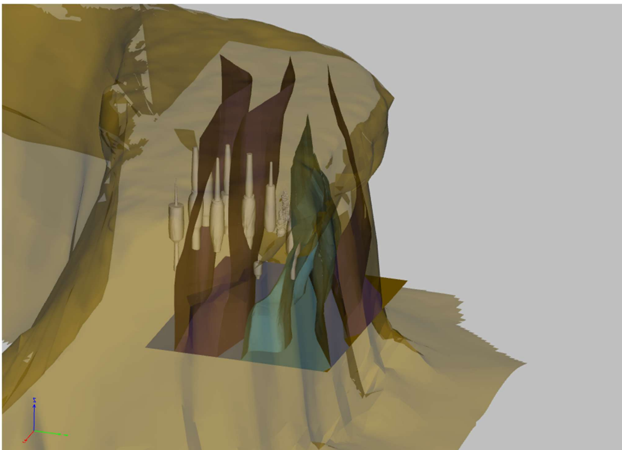
Figuur 5: Voorbeeld uit het 3D geologisch model waarin ook de interne structuur (te zien aan de paarse en blauwe vlakken) van het zoutvoorkomen is weergegeven naast de bestaande cavernes in het veld. Elke nieuwe boring geeft nieuwe informatie over de interne structuur en kan leiden tot aanpassingen van het model. De groene pijl wijst naar het Noorden.
