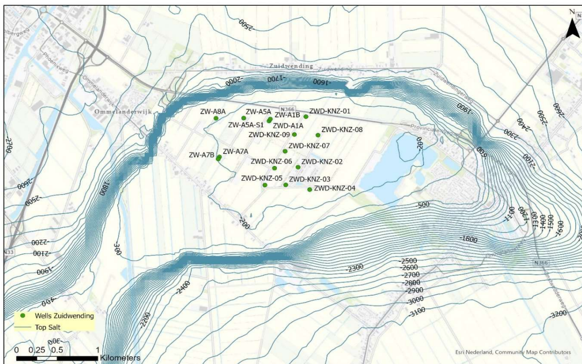
Figuur 1: Overzicht van de putten in het veld in combinatie met dieptecontouren voor het zoutvoorkomen
