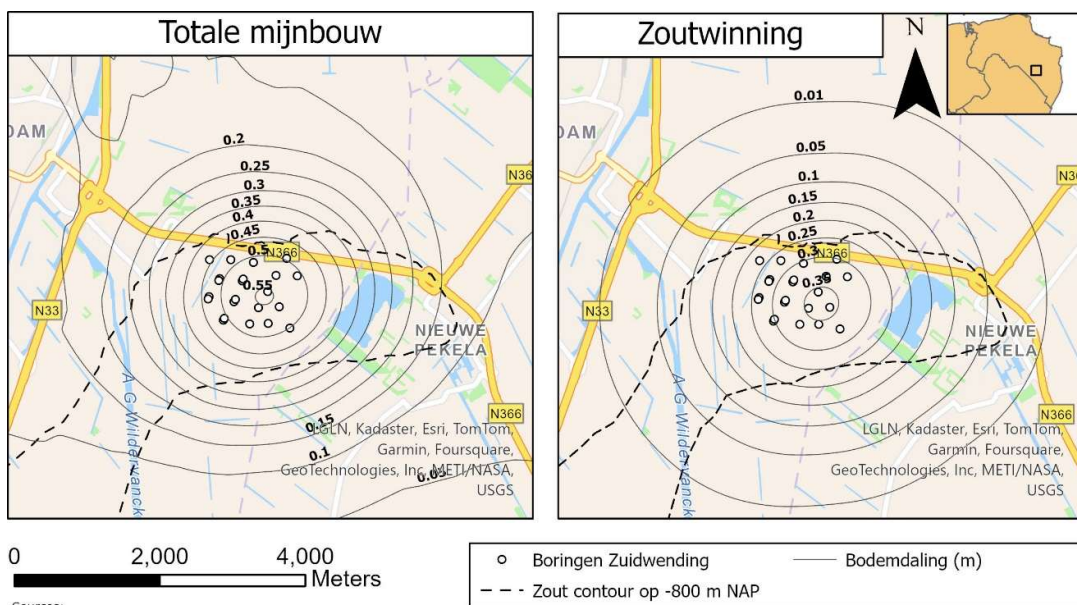
Figuur 25: Bodemdalingsprognose 2200; verwacht scenario.
