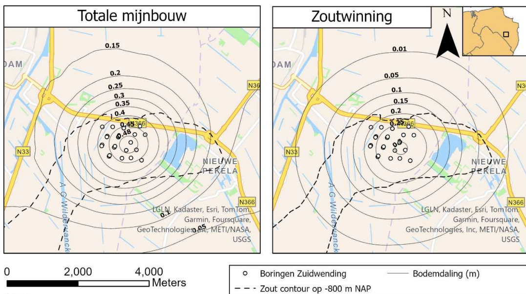
Figuur 23: Bodemdalingsprognose 2150, verwacht scenario
