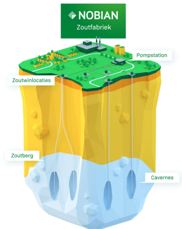
Figuur 7: Illustratie waarin de koppeling tussen caverne en bovengrondse installatie schematisch wordt weergegeven
