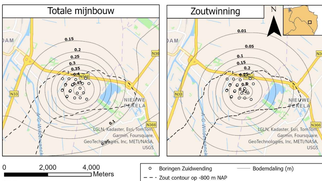
Sources: DEEP.KBB, 2024 Figuur 16: Bodemdalingsprognose 2050; conservatief scenario.
