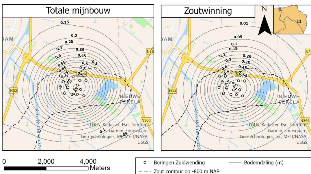
Figuur 22: Bodemdalingsprognose 2125 conservatief scenario
