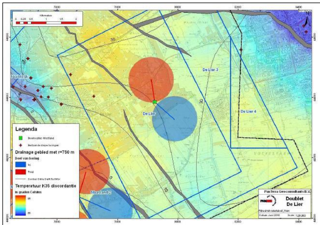
Figuur 4: Breuken in omgeving De Lier (afstand 900m op reservoir niveau).
