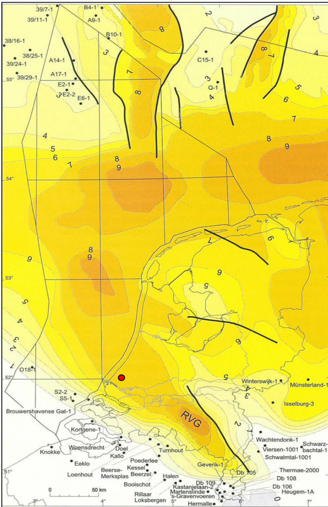
Figuur 3: Schematische dieptekaart in kilometers van de top van de pre-Silezische. Putten die de pre-Silezische zijn tegengekomen zijn aangegeven. Figuur uit Geluk et al. (2007).
