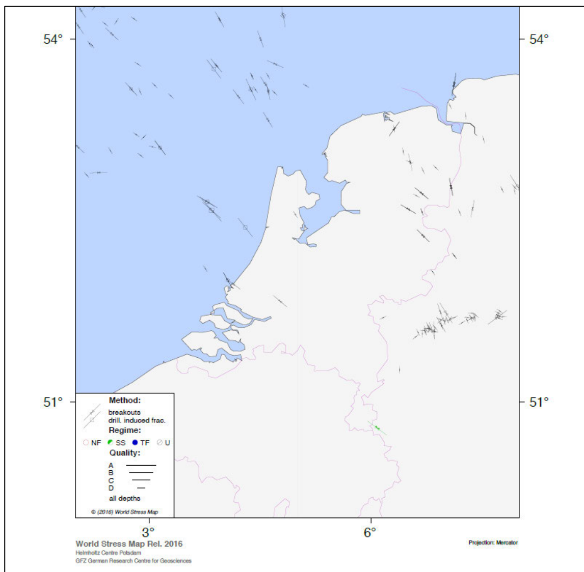
Figuur 5: Oriëntatie Stressveld in Nederland
