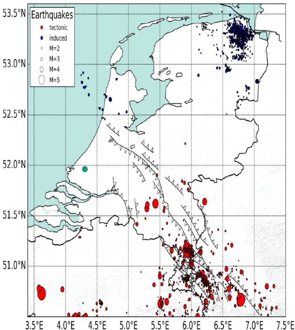
Figuur 6: Natuurlijke (rode) en geïnduceerde (blauwe) seismiciteit in Nederland (KNMI-catalogus vanaf maart-2016, http://cdn.knmi.nl/knmi/map/page/seismologie ). De symboolgrootte wordt geschaald naar aardbevingsgrootte volgens de legenda. Storingstrajecten van het Roer Valley-spiersysteem zijn aangegeven (gegevensbron: Universiteit van Utrecht, 2016).
